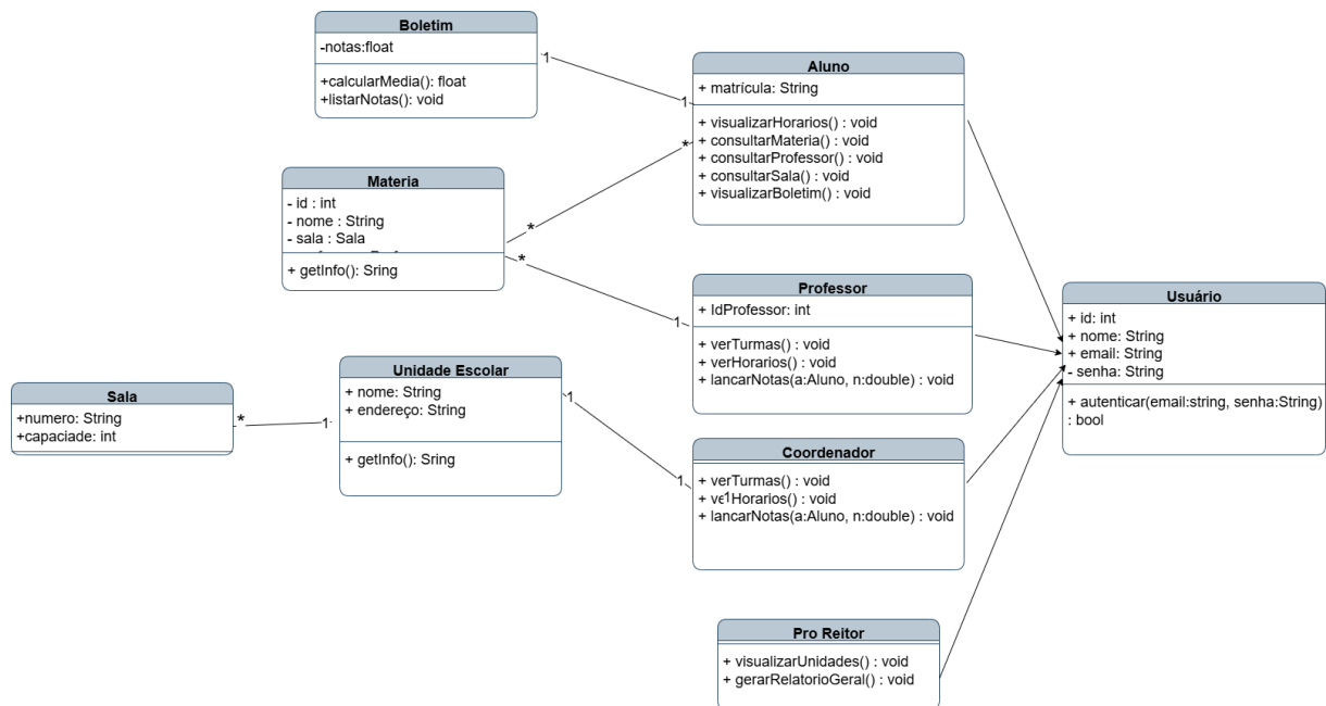
Figura 5.2: Diagrama UML
