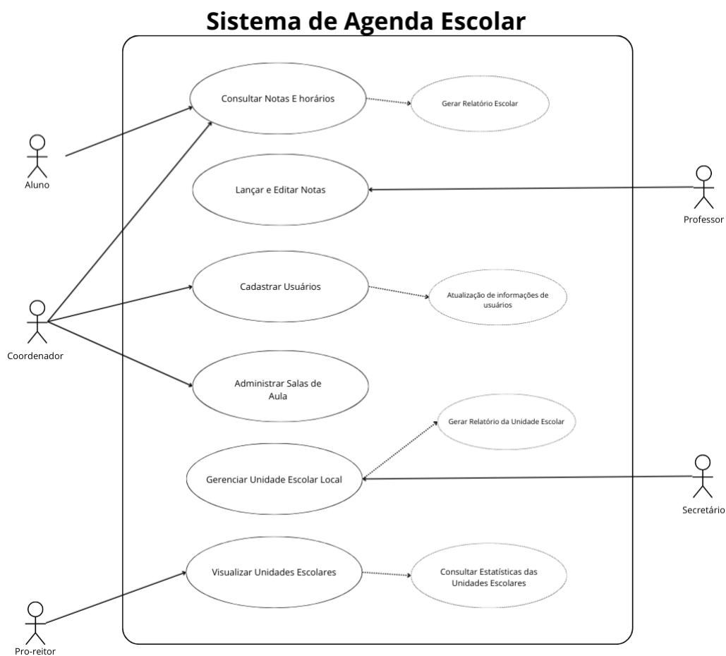
Figura 5.1: Diagrama de Casos de Uso
